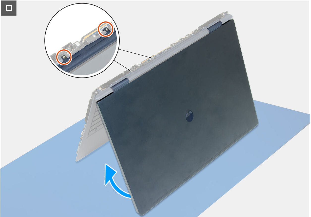
Rakam 66. Orta çubuğu takma
