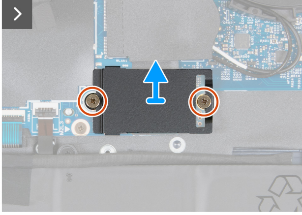
Rakam 30. Resim: M.2 2230 SSD'yi SSD1 yuvasından çıkarma
