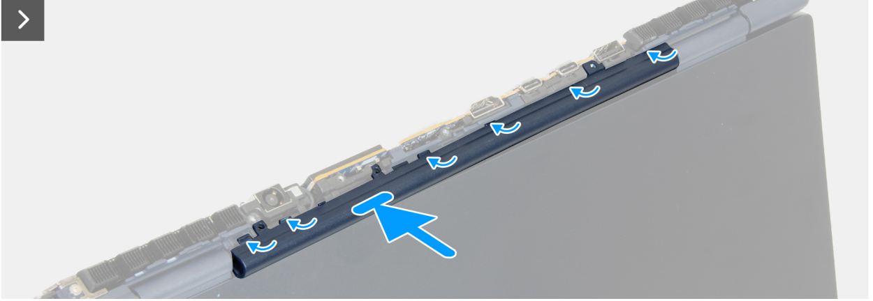
Rakam 65. Orta çubuğu takma
