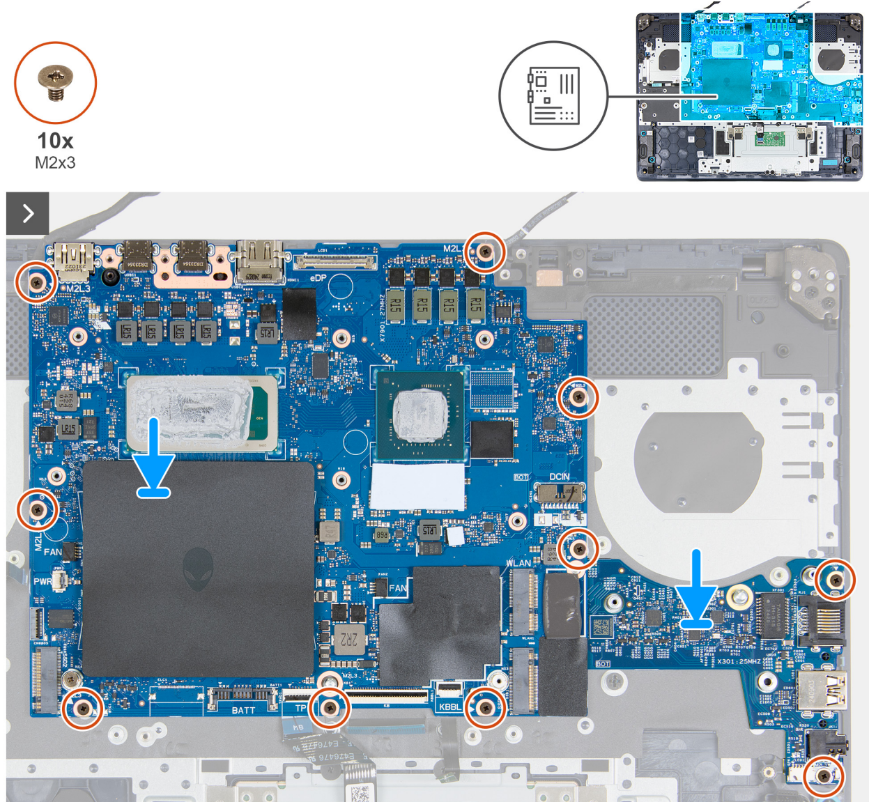
Rakam 56. Sistem kartını takma
