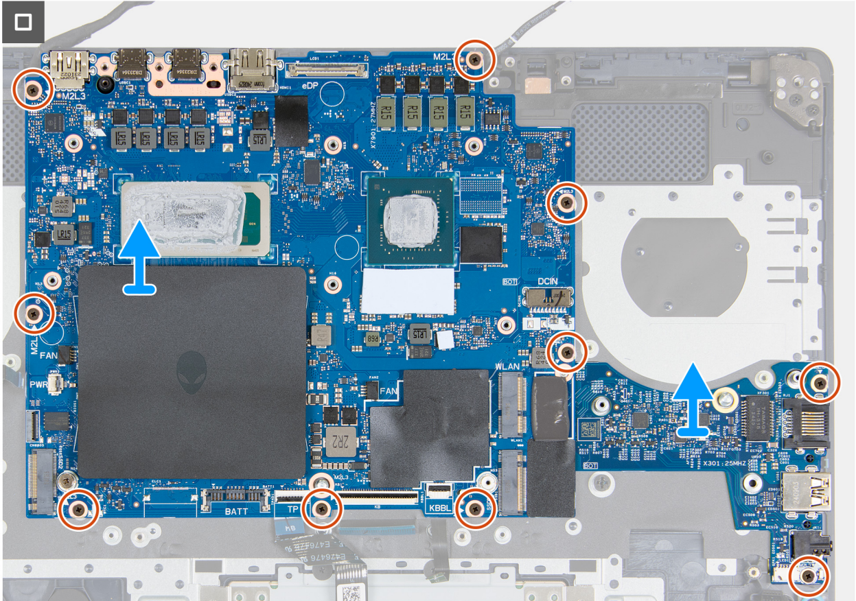
Rakam 54. Sistem kartını çıkarma
