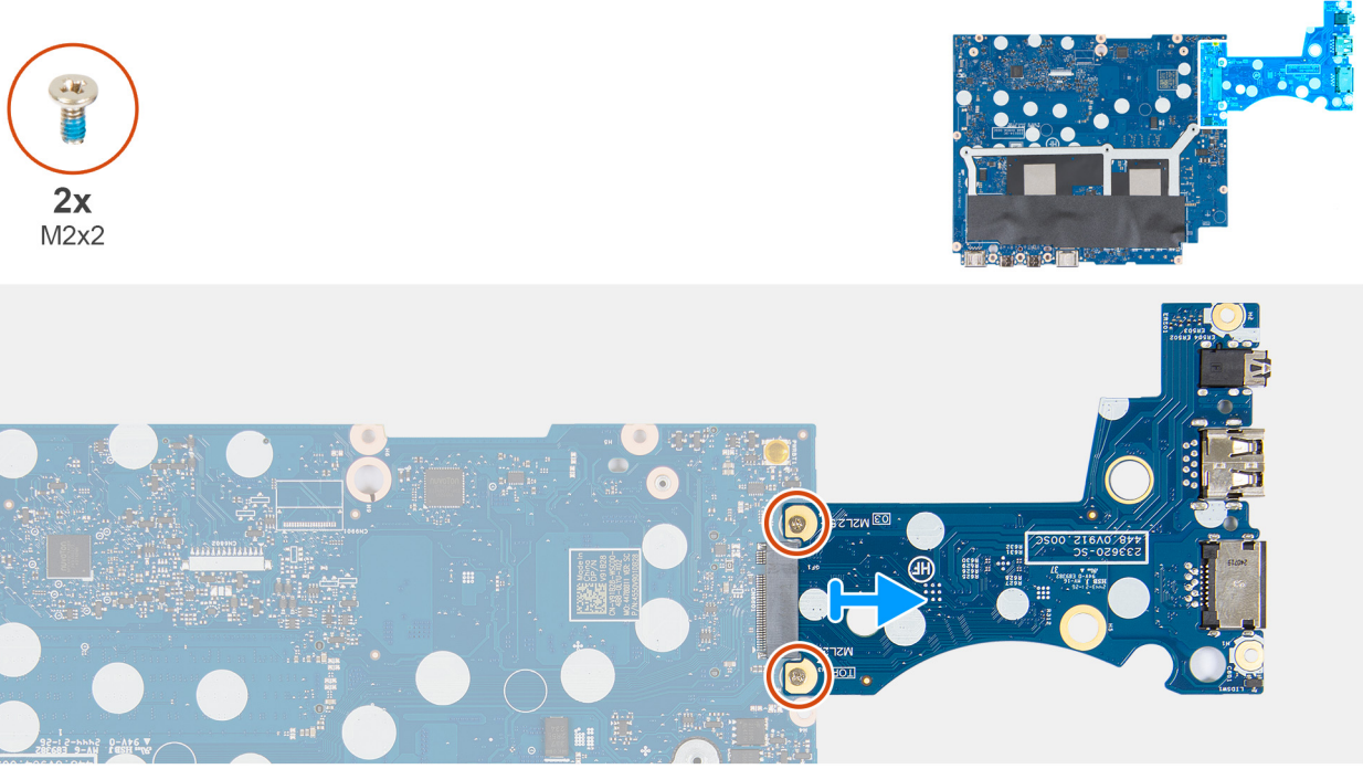
Rakam 58. G/Ç kartını çıkarma
