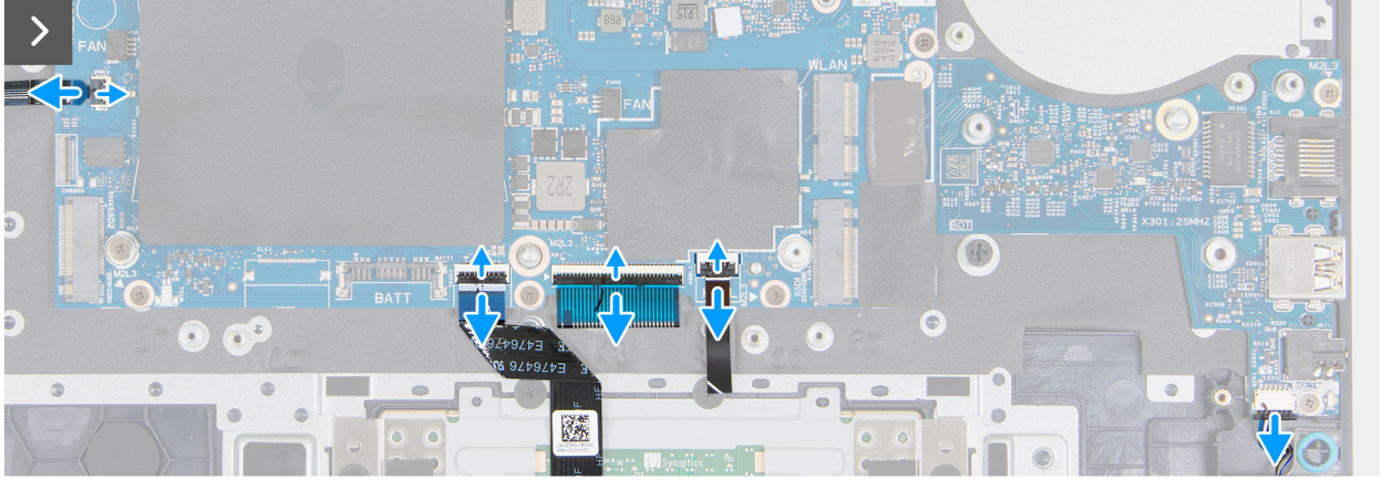
Rakam 53. Sistem kartını çıkarma
