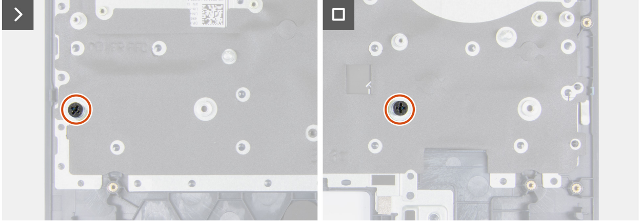
Rakam 74. SSD vida bağlantı parçalarını takma
