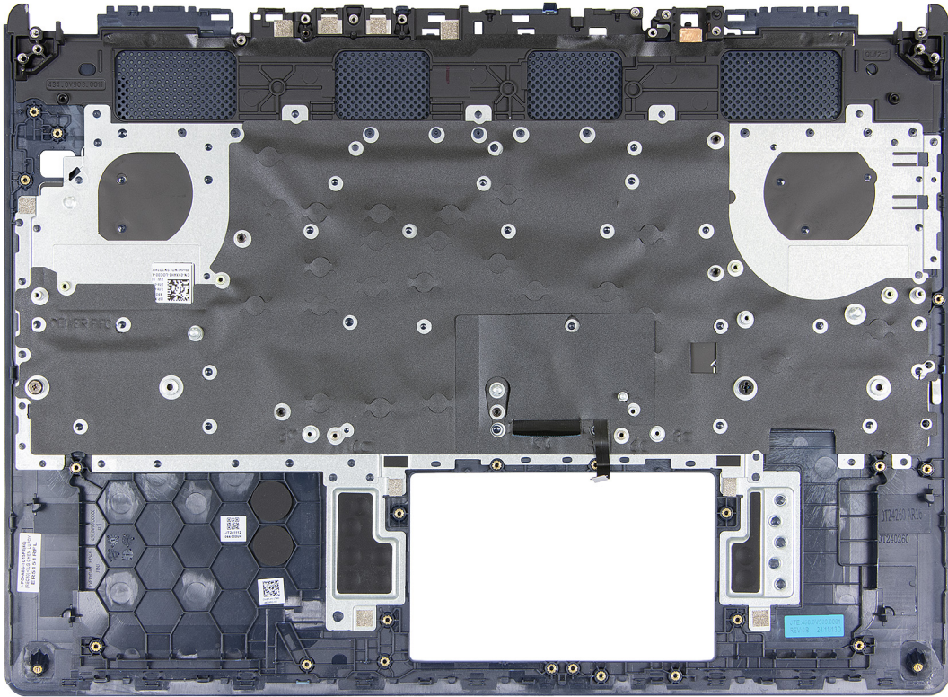
Rakam 75. Avuç içi dayanağı ve klavye aksamını takma
