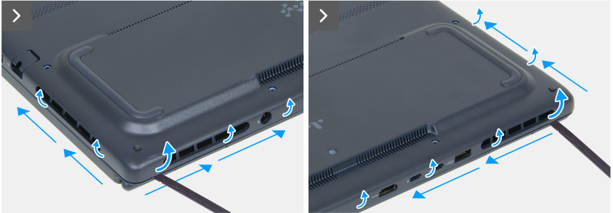
Rakam 13. Yazıcıyı boşluk arasına yerleştirme
