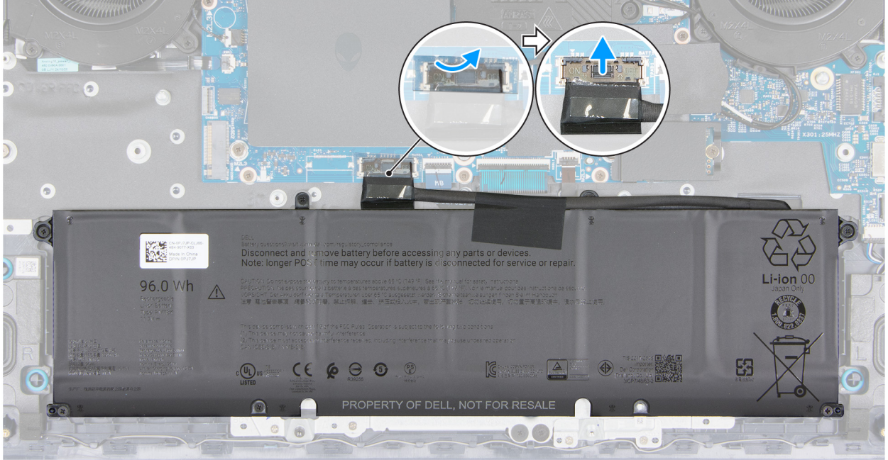
Rakam 15. Pil kablosunu çıkarma
