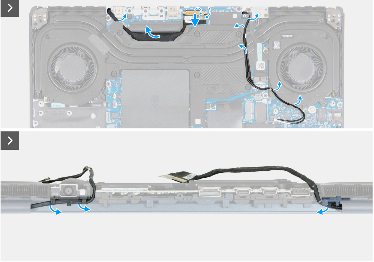
Rakam 67. Ekran aksamını çıkarma
