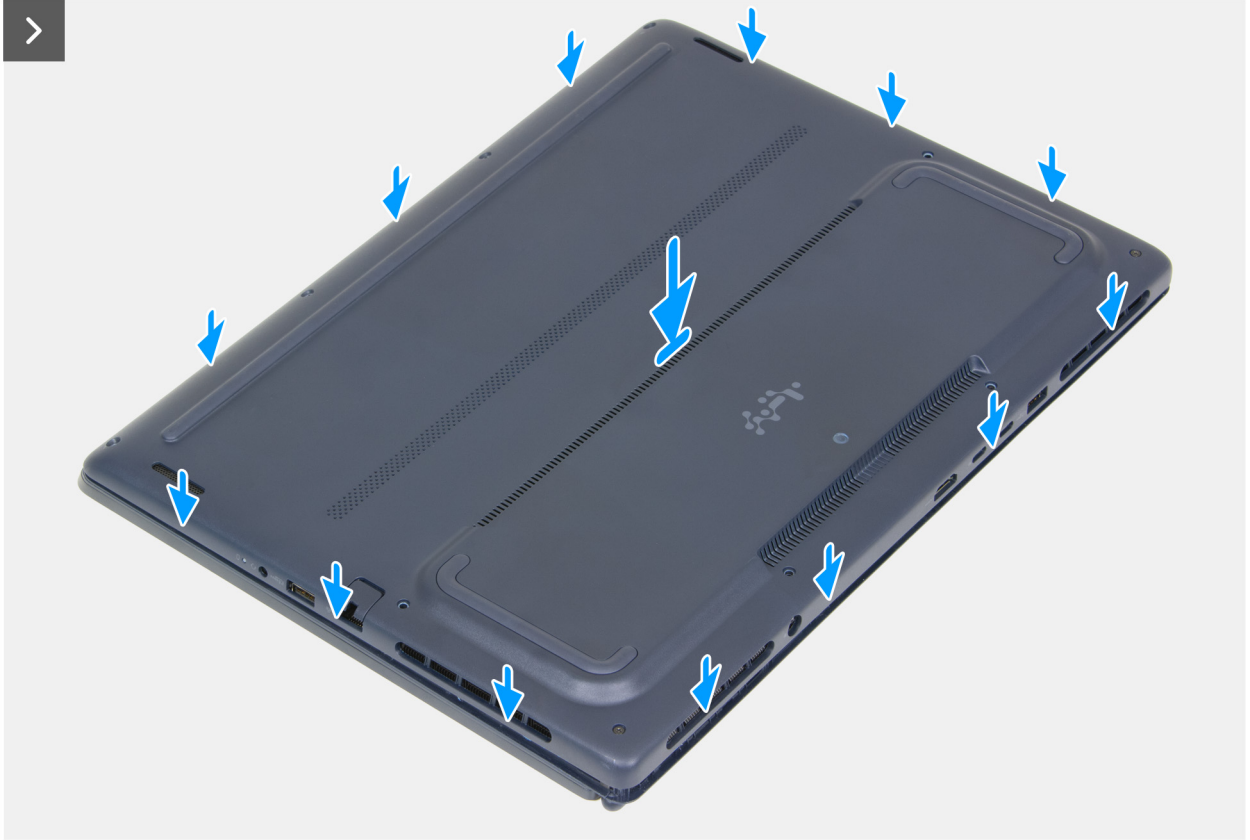
Rakam 18. Alt kapağı takma
