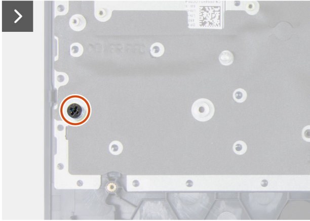
Rakam 73. SSD vida bağlantı parçalarını çıkarma
