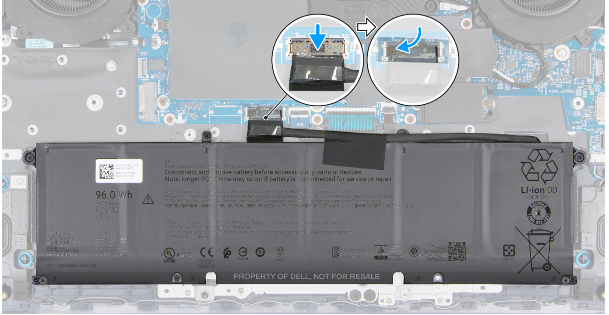
Rakam 17. Pil kablosunu bağlama
